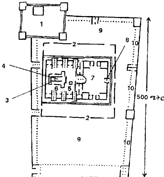
የሄሮድስ ቤተ መቅደስ ንድፍ
