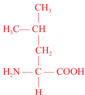
Leucine (Leu, L)
