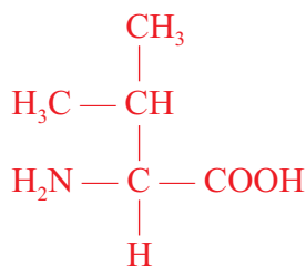
Valine (Val, V)
