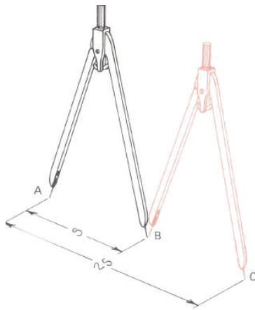
Fig. 2.21 Divider
